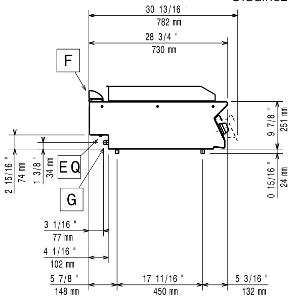
Oldalnézet
